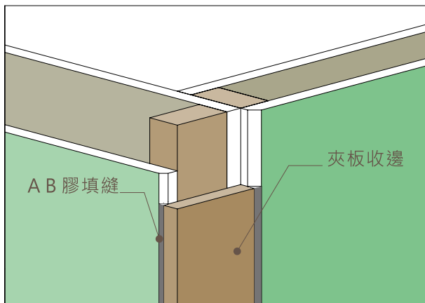
轉角收邊
