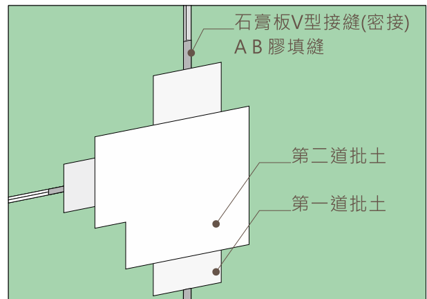
接縫處理
