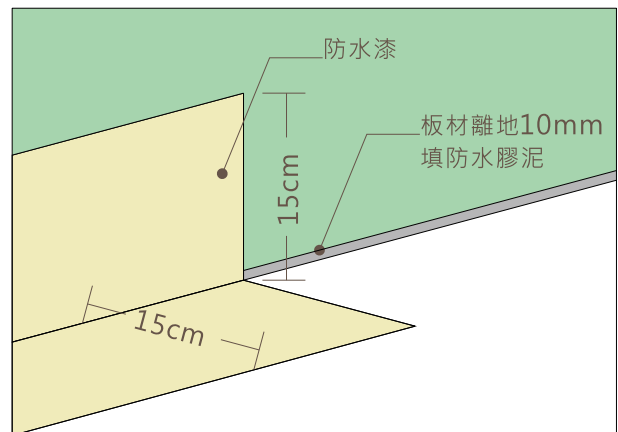
角隅防水
