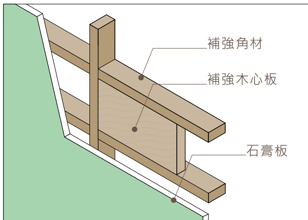
懸掛補強
