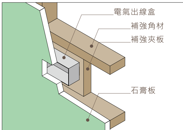
電氣出線盒
